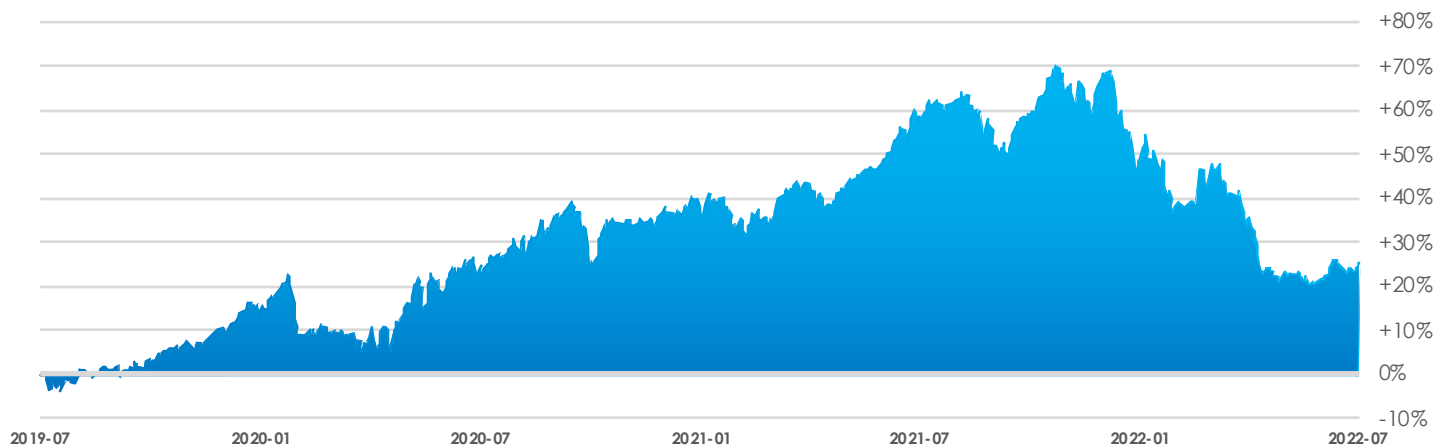
FondNavigator 0-100 Balanserad (+25,3%)
